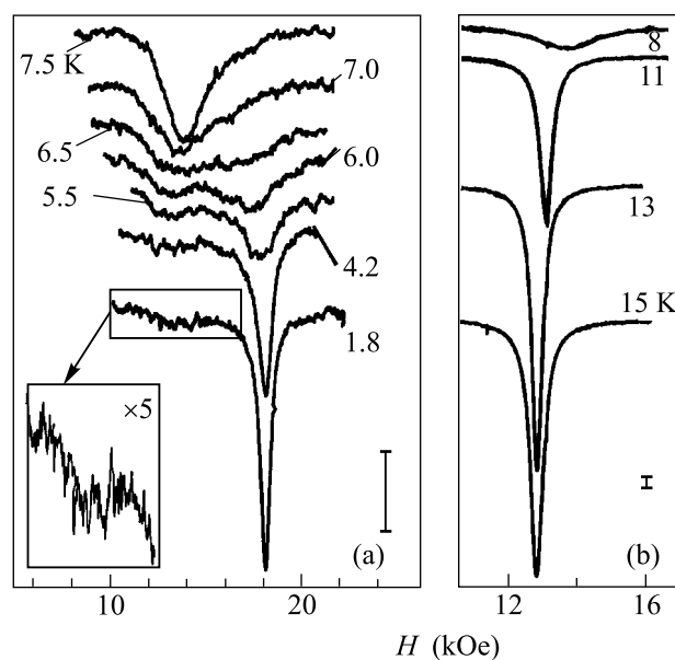
Рис.2. Эволюция формы линии резонансного поглощения образца \text{Cu}_{0.998}\text{Ni}_{0.002}\text{GeO}_3 при изменении температуры [20]. f = 36 ГГц, \mathbf{H} \parallel c , вертикальные отрезки в панелях (a) и (b) соответствуют одинаковой величине поглощения
