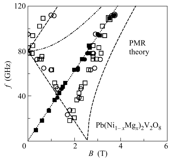
Рис.7. Зависимость резонансной частоты от магнитного поля керамических образцов \text{Pb}(\text{Ni}_{(1-x)}\text{Mg}_x)_2\text{V}_2\text{O}_8 в парамагнитной фазе ( T = 5 К, черные символы) и в упорядоченной фазе ( T = 1.3 К, светлые символы) [25]: x = 0.04 – кружки; x = 0.06 – квадраты
