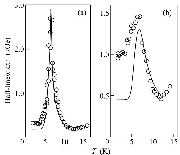
Рис.5. Зависимость ширины линии ЭПР от температуры для образцов \text{CuGeO}_3 с x=0.2\% (а) и x=0.8\% (б). Сплошные линии – теоретический расчет [20]
