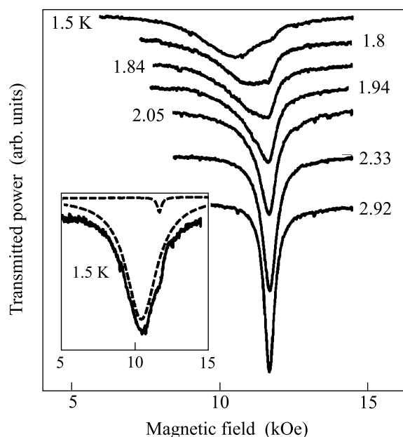
Рис.8. Изменение формы линии магнитного резонанса в окрестности температуры Нееля в монокристалле \text{Cu}_{0.983}\text{Mg}_{0.017}\text{GeO}_3 [27]: \mathbf{H} \parallel b , f = 36 ГГц, T_N = 2.25 К
