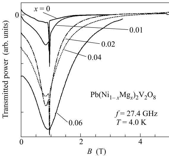
Рис.6. Линии магнитного резонанса разбавленного халдейновского магнетика, нормированные на единицу массы [25]. Узкая линия при B = 0.98 Тл – метка дифракции полиакриламидгидразила: g = 2.0
