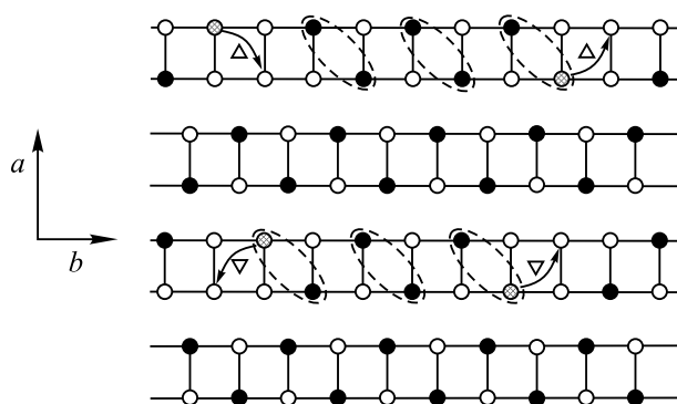
Рис.10. Зигзаговые спиновые цепочки на “лестницах” обменно связанных ионов ванадия в слоях V–O кристаллов \text{NaV}_2\text{O}_5 [32]. Сплошные линии – пути обменного взаимодействия между ионами ванадия, ● – магнитные ионы \text{V}^{4+} , ○ – немагнитные ионы \text{V}^{5+} , серые кружки обозначают ионы ванадия с прыгающими электронами, \Delta -вакансия Na (находится над или под слоем V–O). Стрелками обозначены возможные прыжки электронов, меняющие четность фрагментов. Пунктирные овалы обозначают димеризацию (альтернирование) цепочек
